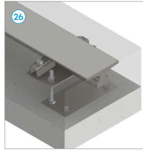
Laufschiene
