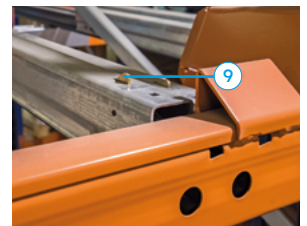
Sicherheitsklinke
