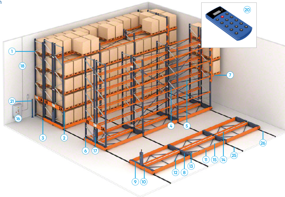
Führungsschiene
